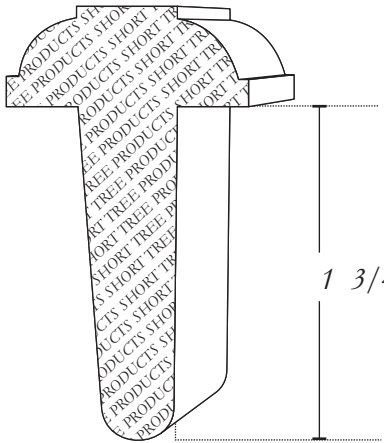
*1 3/4" T-ASTRAGAL
